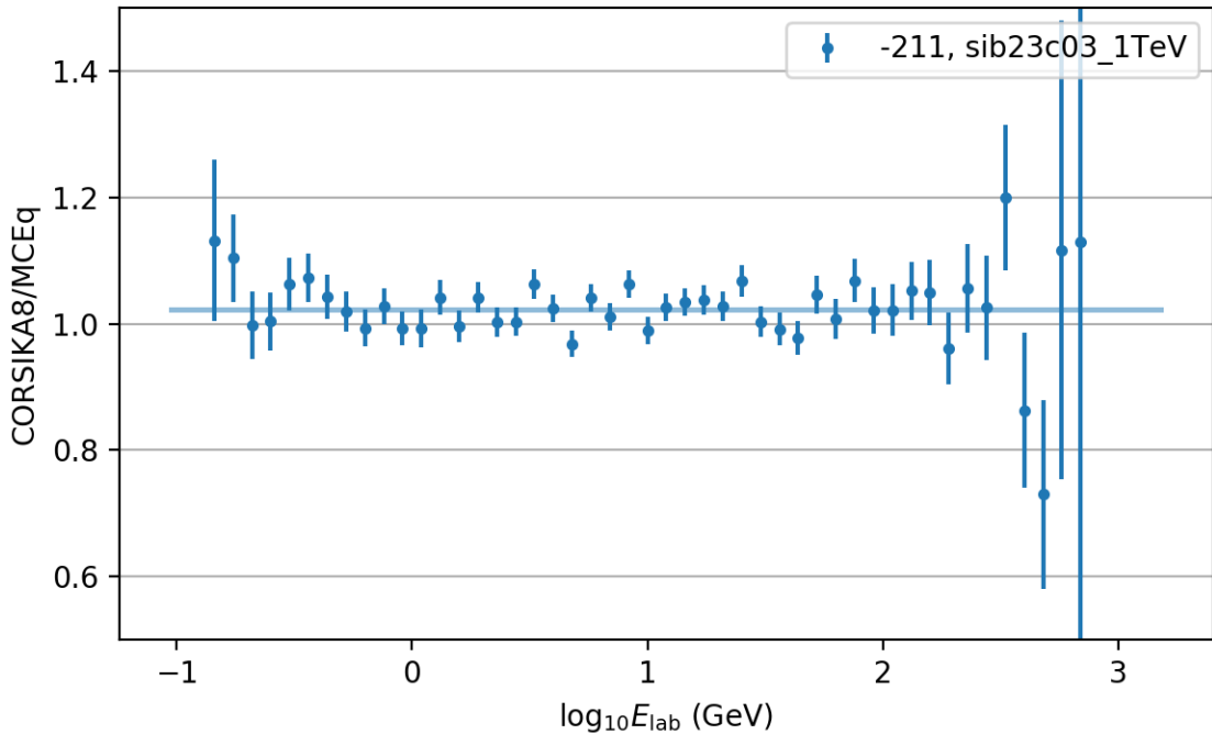
sib23c03_1TeV
