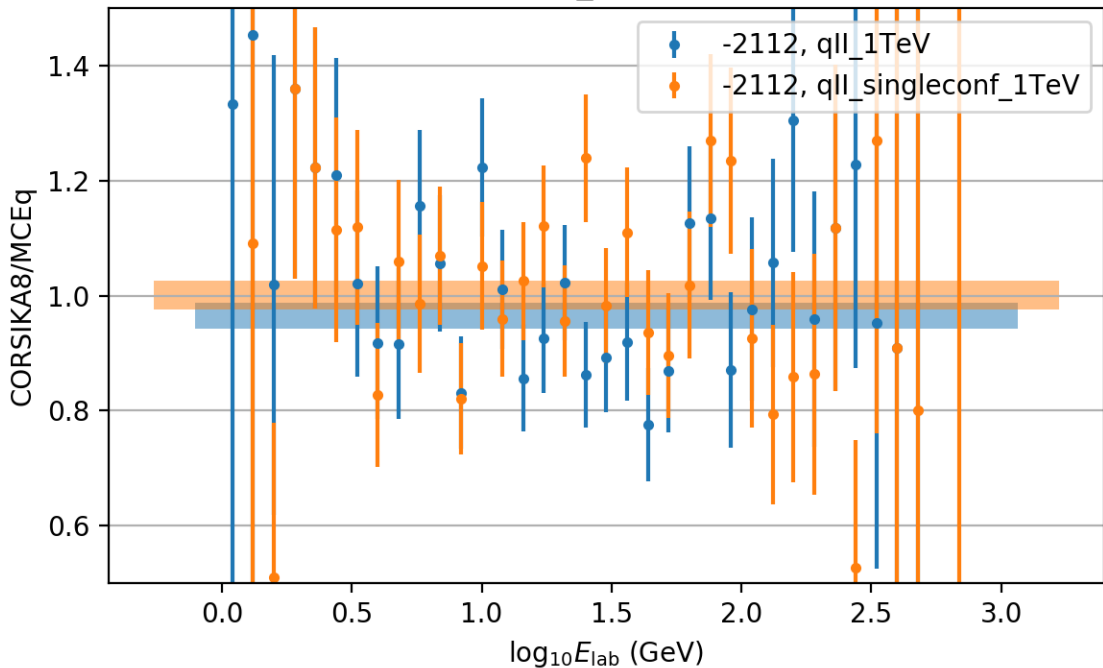
qll_1TeV
