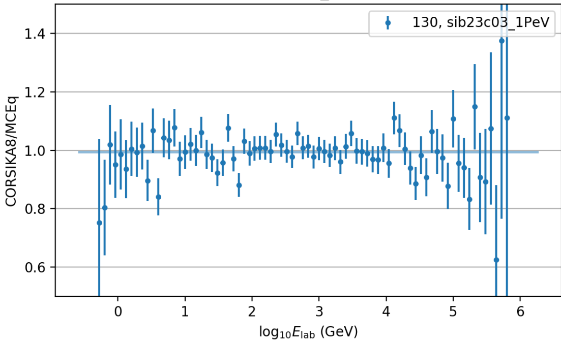
sib23c03_1PeV
