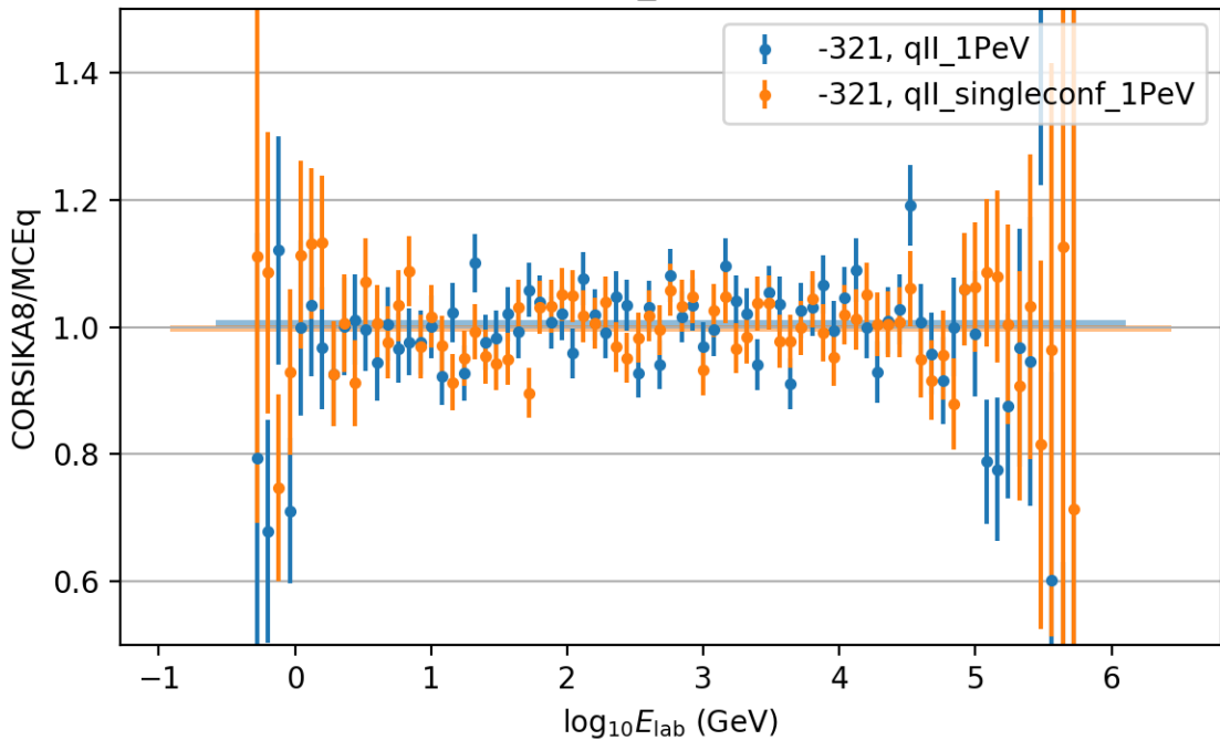
qll_1PeV
